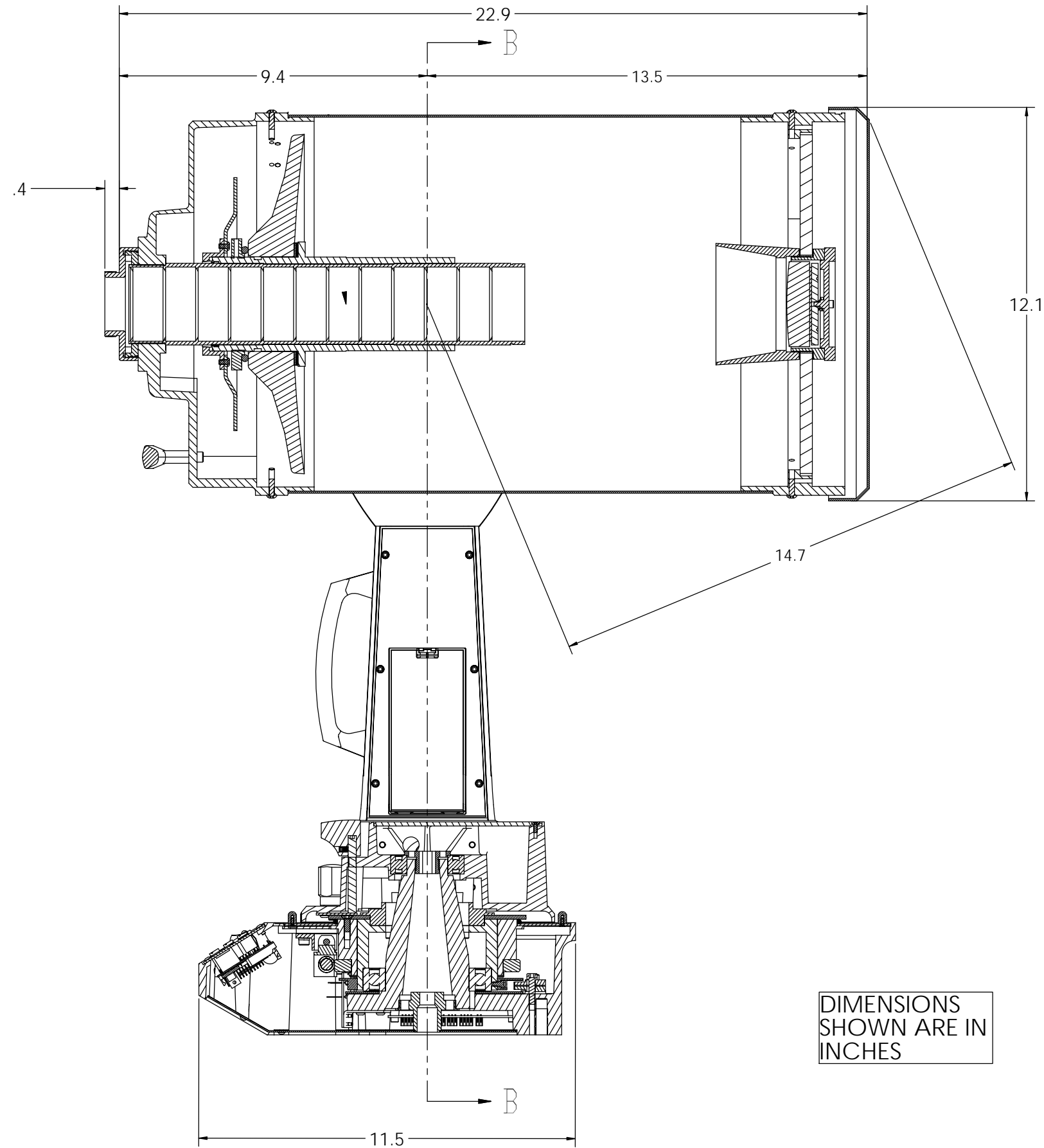
SECTION A-A
